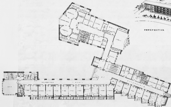
PLANTA PRIMERA
