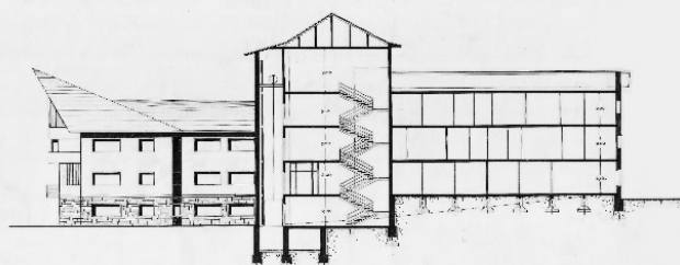
ALZADO SECCION E-F
